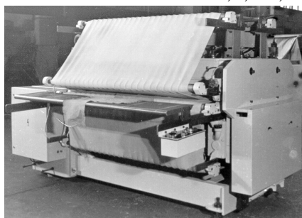
Тянульная машина МОЛЛИСА 1500 мм - габариты 2800x2200x1700 мм
