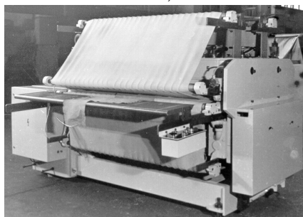
Тянульная машина МОЛЛИСА 1800 мм - габариты 3220x2200x1700 мм
