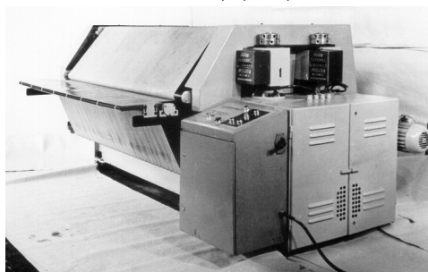
Тянульная машина МОЛЛИСА автоматическая 2100 мм - габариты 3410x2200x1750 мм
