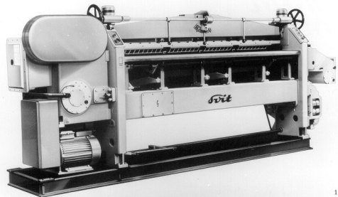
Двоильная машина 3000 мм - габариты 5100x900x1940 мм
