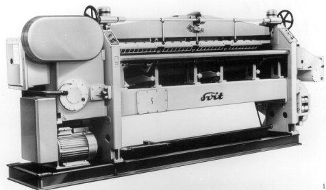
Двоильная машина 1800 мм - габариты 3900x900x1840 мм
