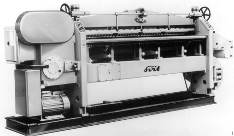
Двоильная машина 2700 мм - габариты 4800x900x1840 мм
